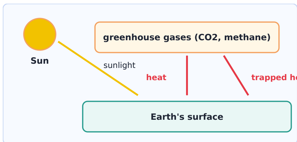
Esquema simplificado do efeito estufa.
